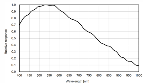
MV-CE200-10UM 量子效率
